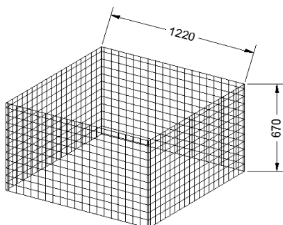
PREFAKOM-1000 1000 litrů
